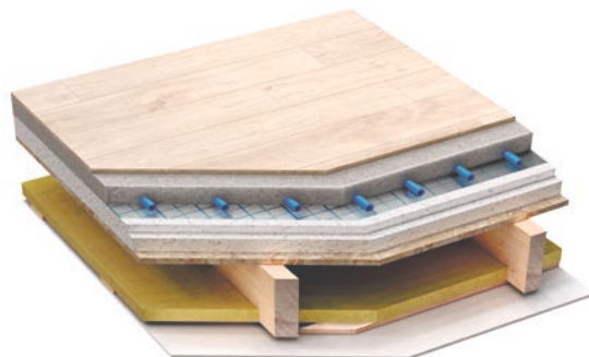
Schema Geschossdecke
