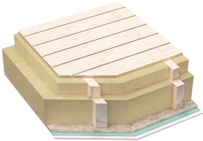
Aufbau der Kehlbalckendecke zum unbeheizten Spitzboden
