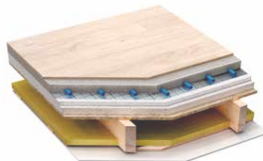
Schema Geschossdecke
